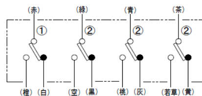
接点構成 4c
