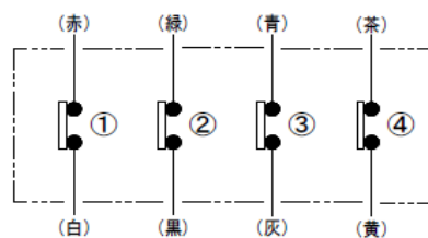
接点構成 4b
